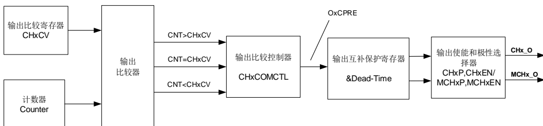
图 23-102. 输出比较逻辑（x = 1）
