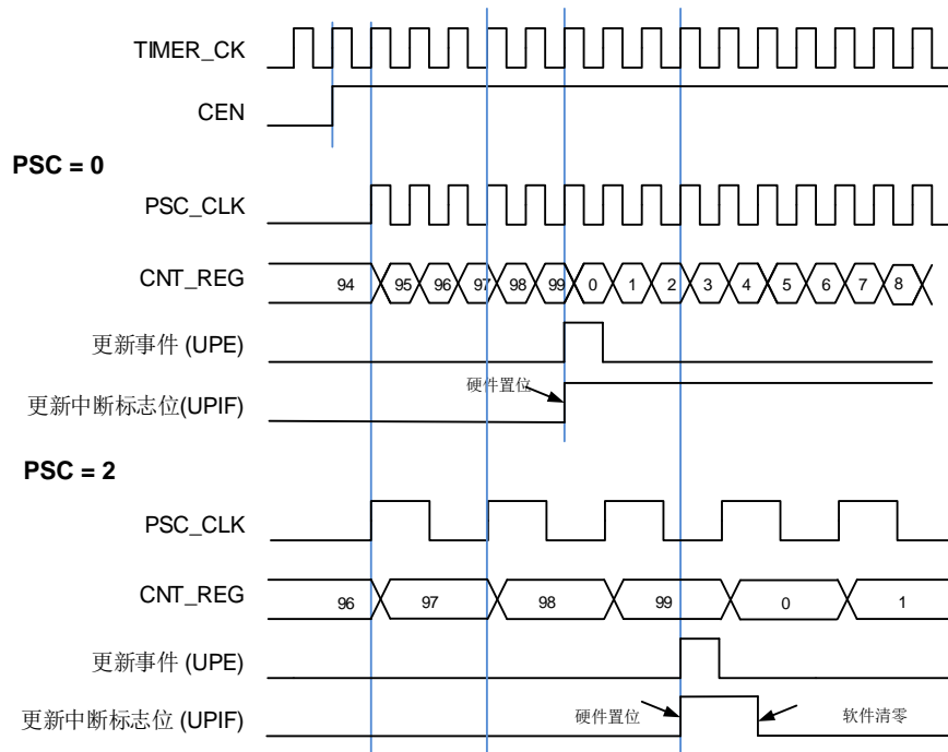
图 23-126. 向上计数时序图, PSC = 0 / 2
