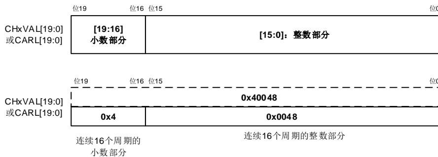
图 23-105. 微调模式: 数据格式和寄存器位域
