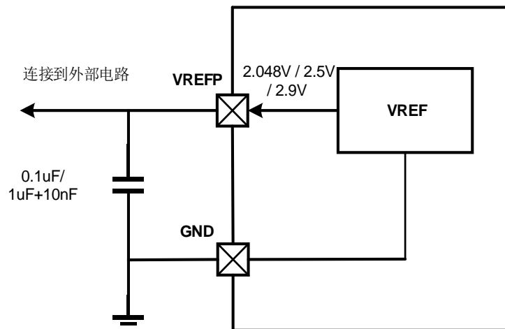
图 20-1. VREF 连接
