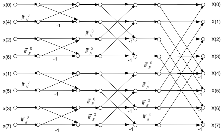
图 15-2. 8 点 DIF 的 FFT 流程图
