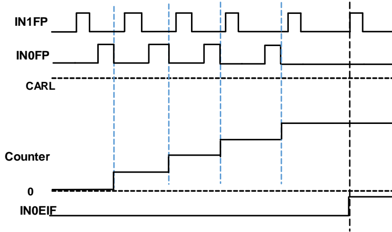
图 24-15. 计数器运行在编码器模式 1 (同相, IN0EIF)
