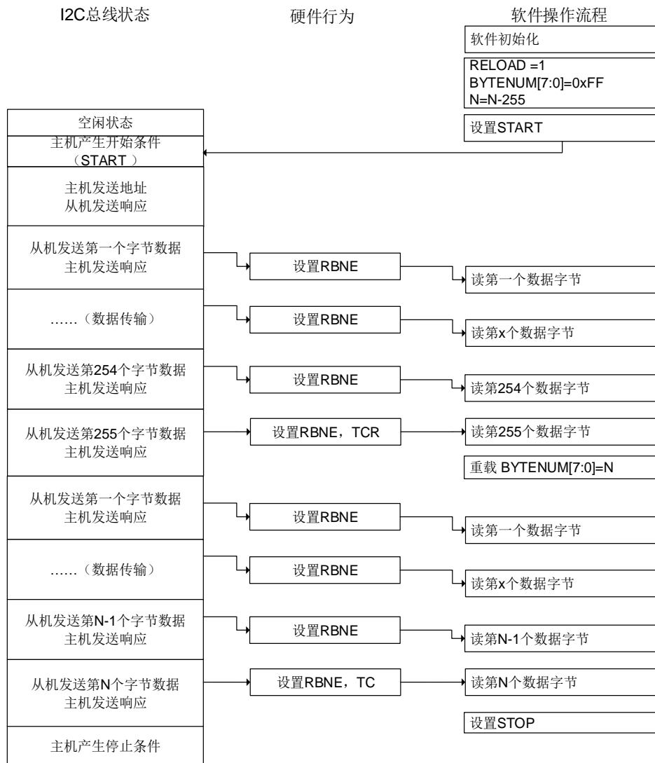
图 28-21. I2C 主机接收编程模型 (N>255)
