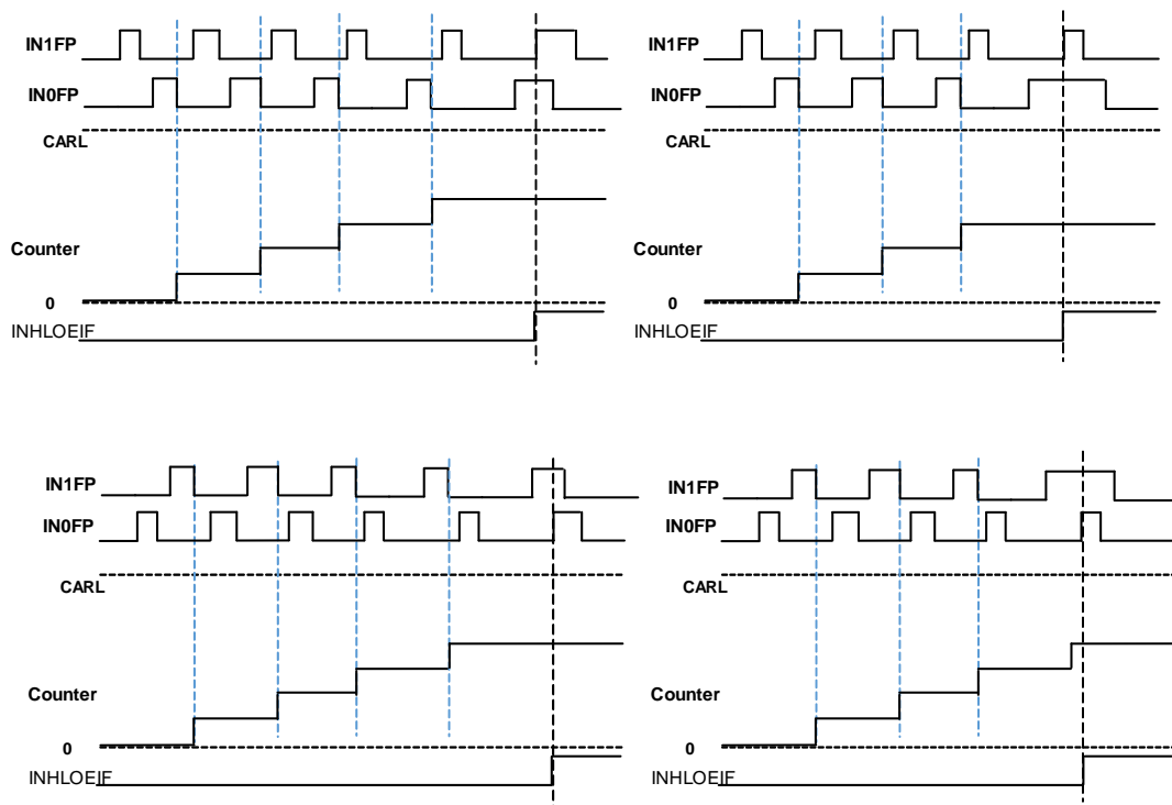
图 24-17. 计数器运行在编码器模式 1（同相，INHLOEIF）
