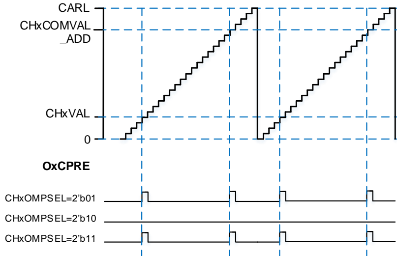
图 23-27. 边沿对齐模式下 CHx_O 输出脉冲 (CHxOMPSEL ≠ 2'b00)
