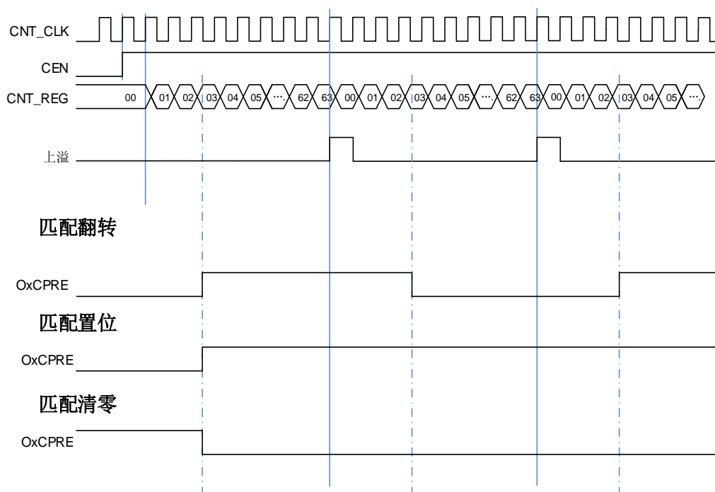
图 23-103. 三种输出比较模式
