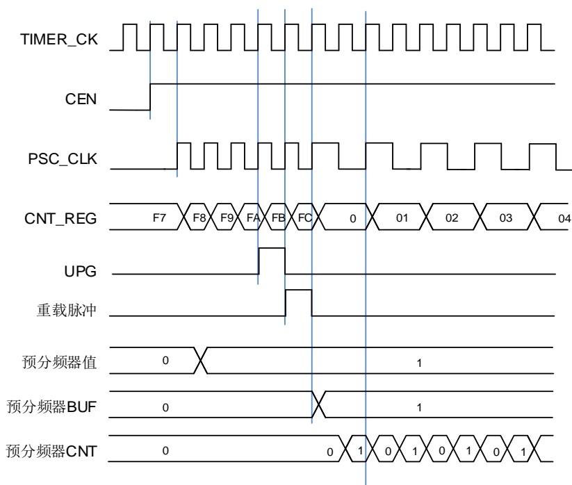
图 23-125. 当预分频器的参数从 1 变到 2 时, 计数器的时序图
