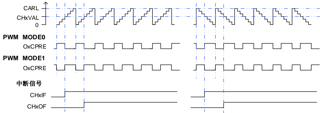
图 23-76. CAPWM 时序图
