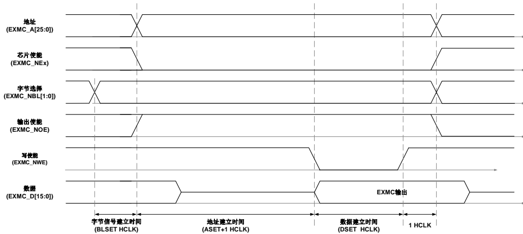
图 33-5. 模式 1 写时序
