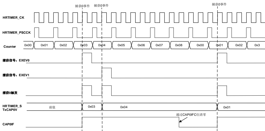
图 25-11. EXEV0 和 EXEV1 触发捕获 0
