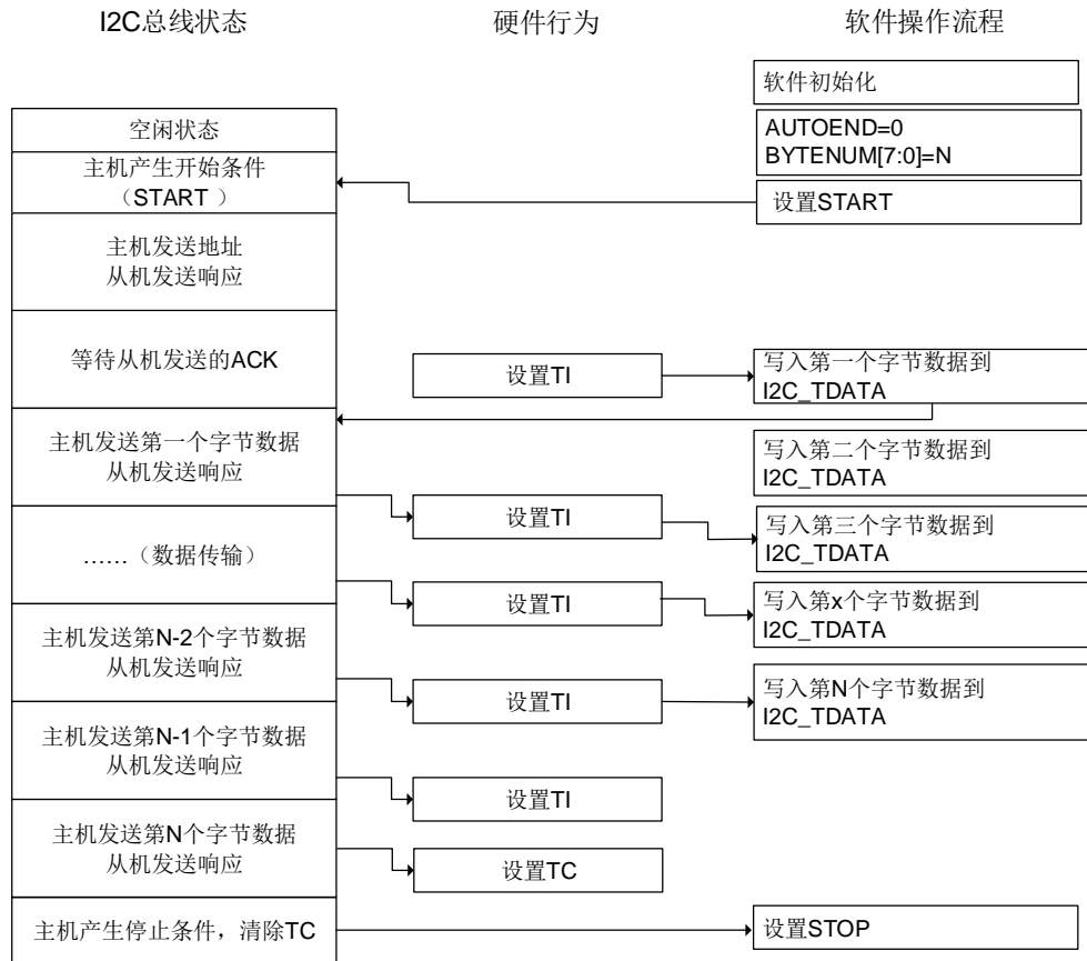
图 28-18. I2C 主机发送编程模型 (N<=255)
