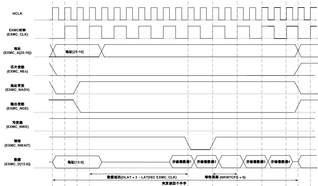
图 33-19. 同步复用突发传输读时序
