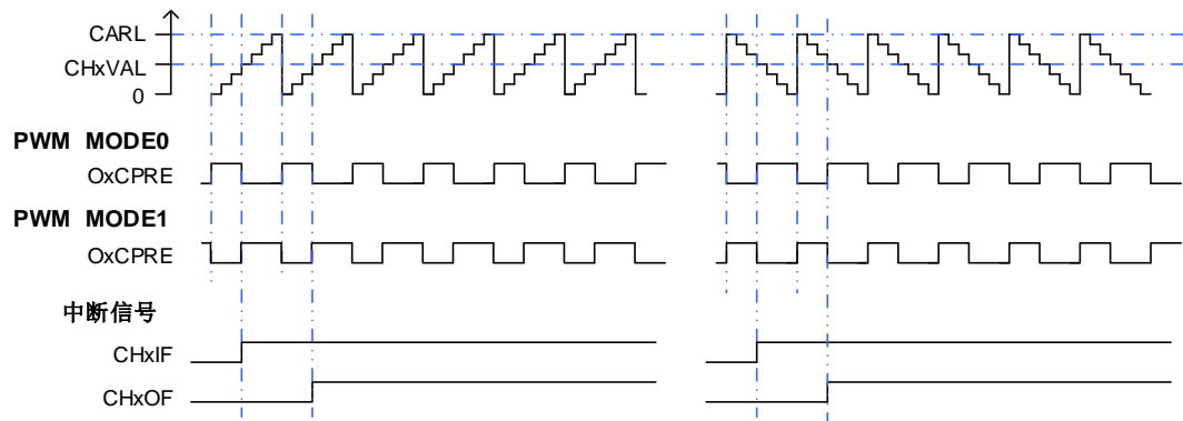
图 23-18. CAPWM 时序图
