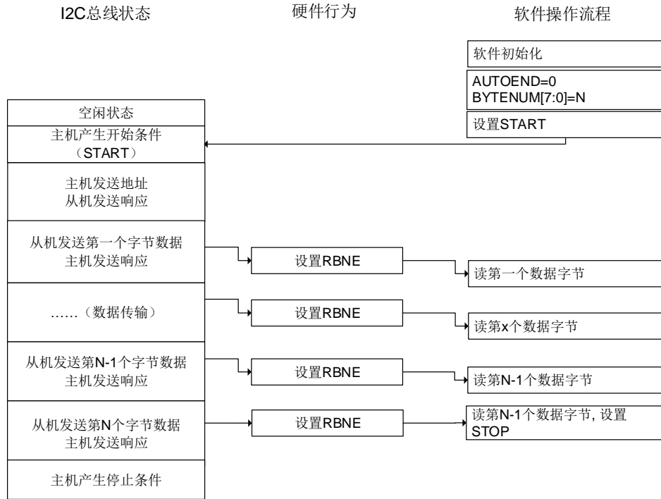
图 28-20. I2C 主机接收编程模型 (N<=255)
