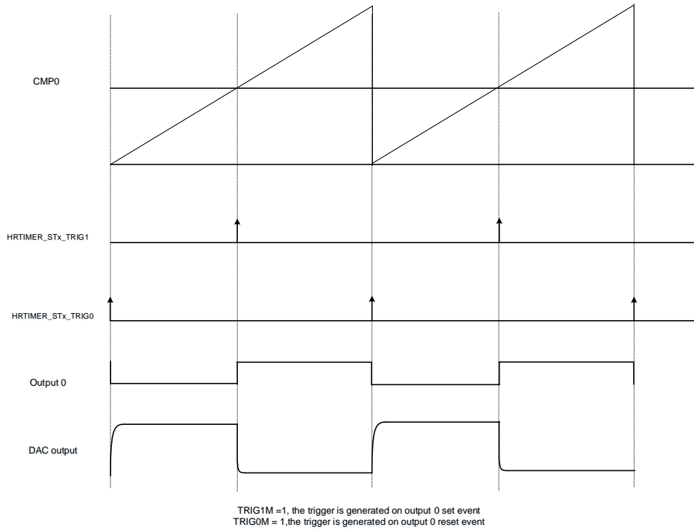
图 25-58. 当 TRIG0M = 1 和 TRIG1M = 1 时 DAC 触发
