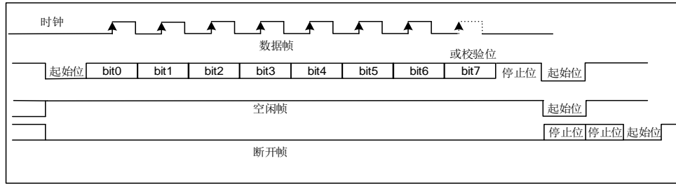
图 27-2. USART 字符帧（8 数据位和 1 停止位）
