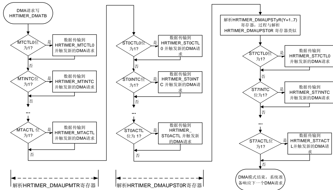
图 25-59. DMA 模式运行流程图
