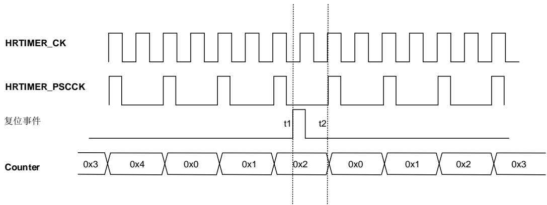
图 25-9. 当预分频系数为 128 时，复位事件重新同步
