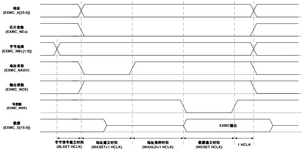
图 33-14. 模式 D 写时序
