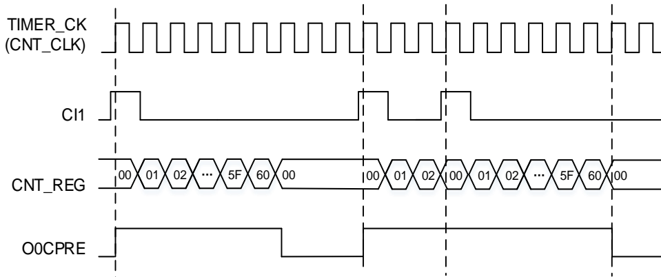
图 23-52. 可延时单脉冲模式 (TIMERx_CHxCV = 0x00, TIMERx_CAR = 0x60)
