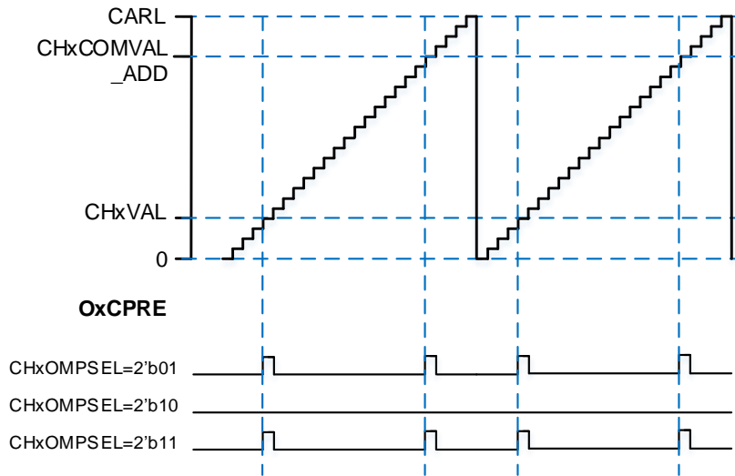
图 23-85. 边沿对齐模式下 CHx_O 输出脉冲 (CHxOMPSEL ≠ 2'b00)
