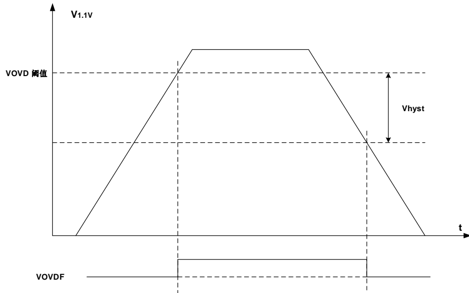
图 3-9. VOVD 波形
