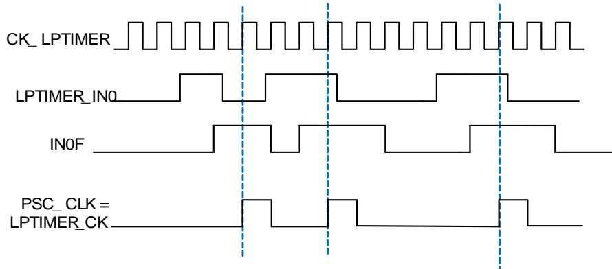
图 24-3. 内部时钟模式 1（CKSSEL = 0, CNTMEN = 1, PSC[2:0] = 000）
