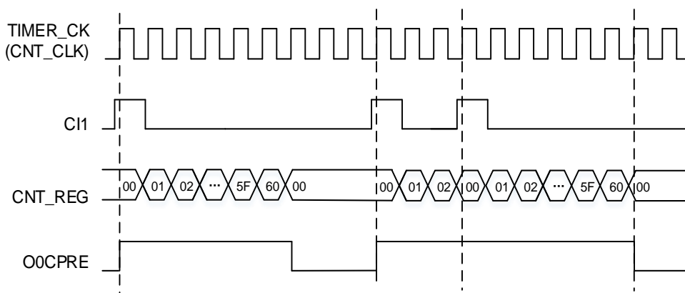
图 23-91. 可延时单脉冲模式（TIMERx_CHxCV = 0x00，TIMERx_CAR = 0x60）
