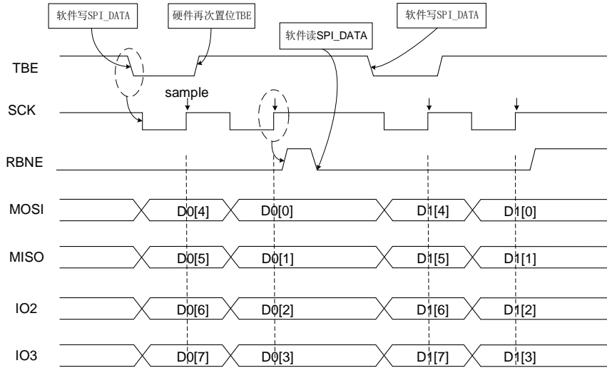
图 30-15. SPI 四线模式读操作时序图
