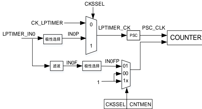
图 24-2. LPTIMER 时钟源选择
