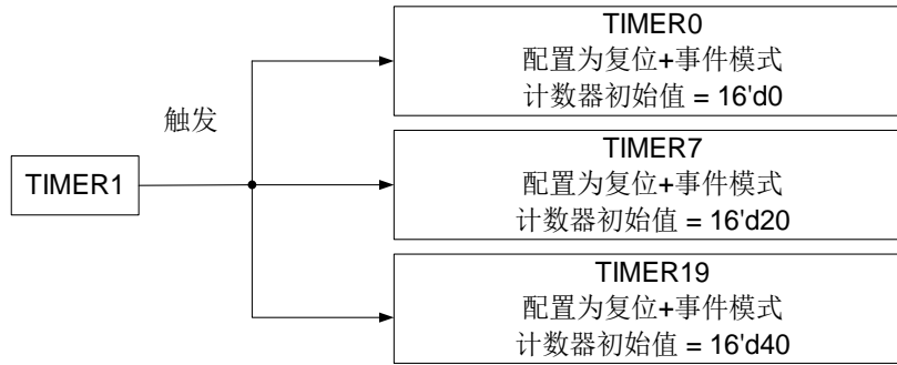
图 23-61. 配置相移方法的框图
