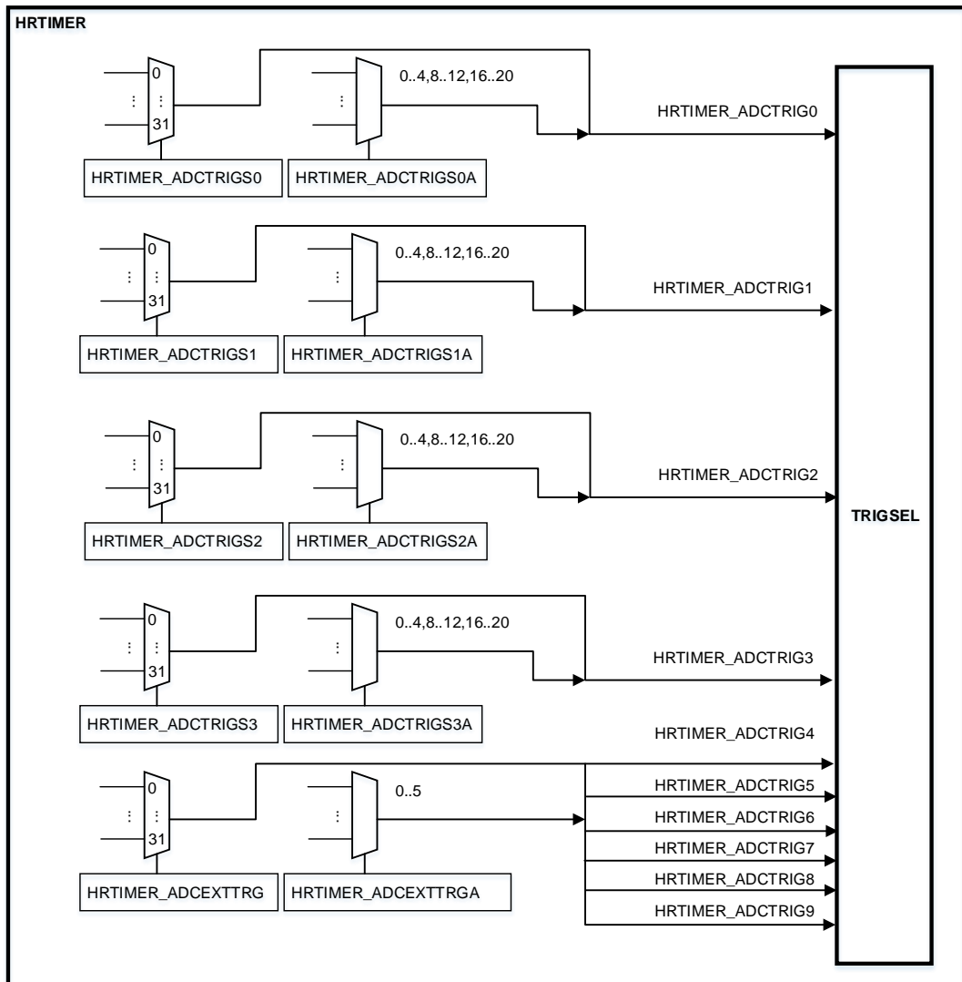
图 25-53. ADC 触发源选择图
