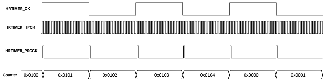
图 25-3. 分频为 32 时计数器时钟
