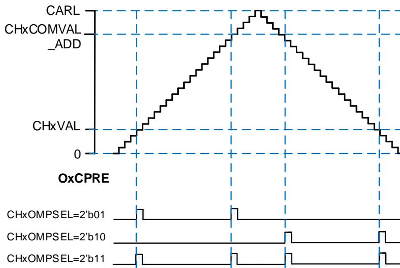
图 23-86. 中央对齐模式下 CHx_O 输出脉冲 (CHxOMPSEL ≠ 2'b00)
