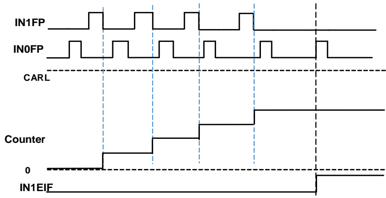
图 24-14. 计数器运行在编码器模式 1（同相，IN1EIF）
