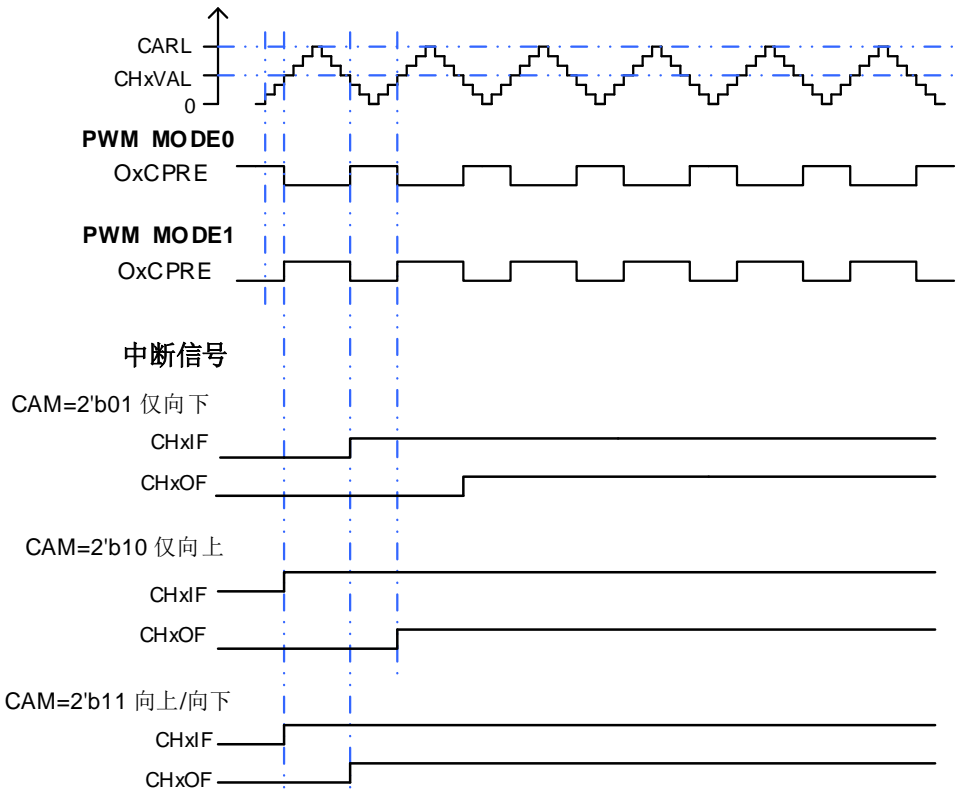
图 23-76. CAPWM 时序图
