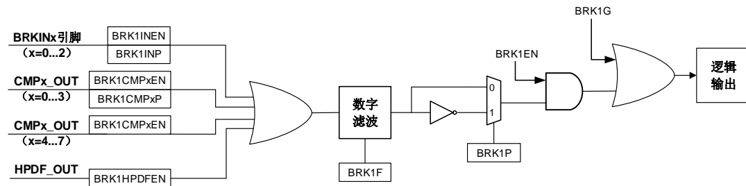
图 23-32. BREAK1 中止功能逻辑图
