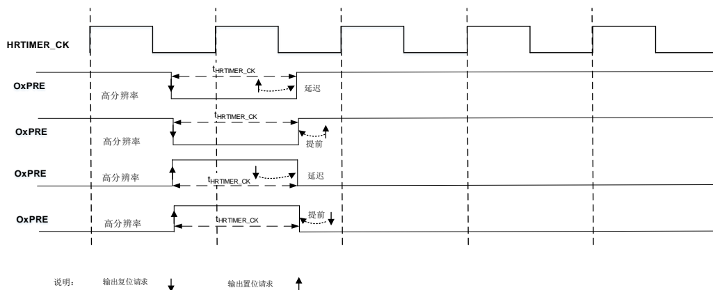
图 25-25. 脉冲宽度为 1 个 t_{HRTMER\_CK} 周期
