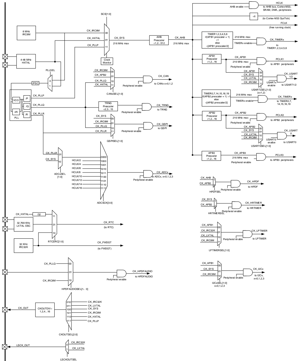
图4-2. 时钟树
