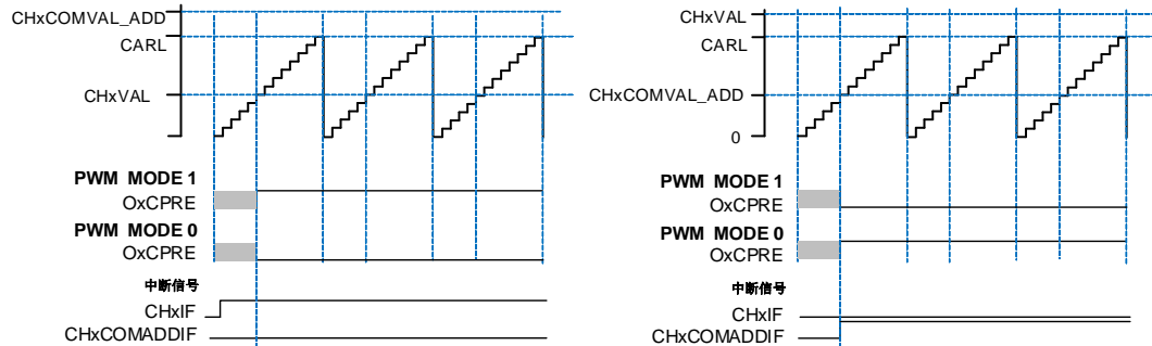
图 23-82. 通道 x 输出 PWM (CHxVAL 或 CHxCOMVAL_ADD > CARL)
