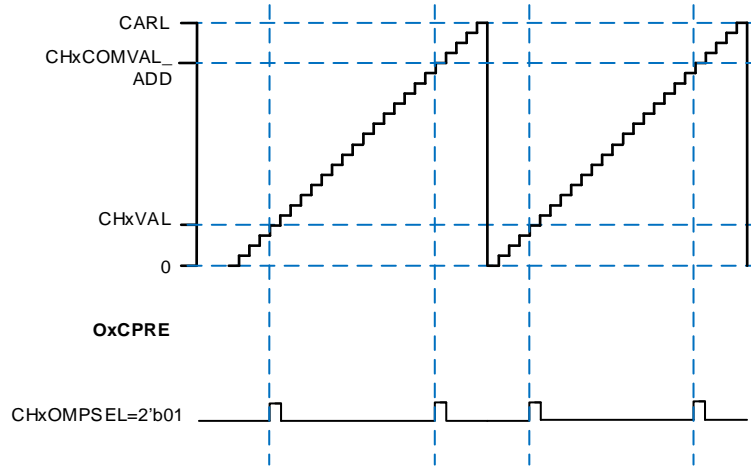
图 23-112. 边沿对齐模式下 CHx_O 输出脉冲 (CHxOMPSEL = 2'b01)
