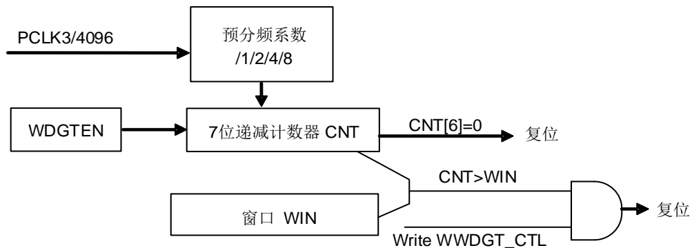
图 21-2. 窗口看门狗定时器框图
