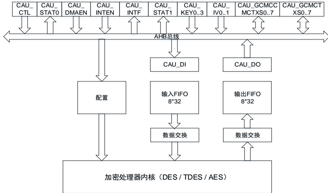
图 13-3. CAU 框图
