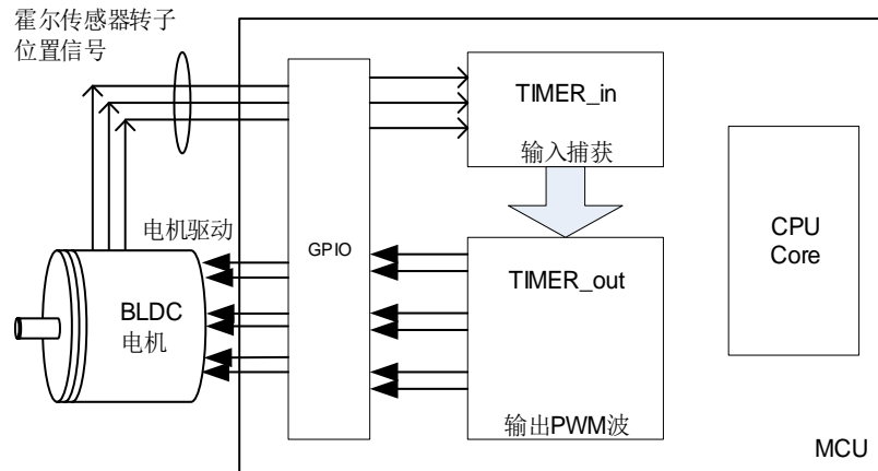
图 23-46. 霍尔传感器用在 BLDC 电机控制中
