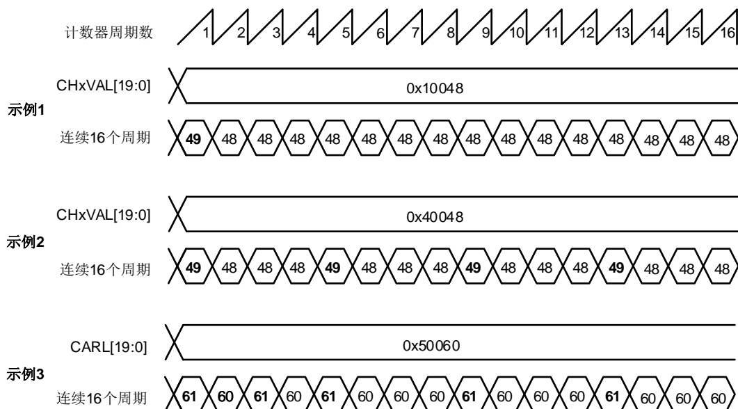
图 23-147. PWM 微调模式原理
