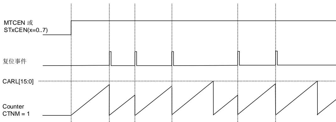
图 25-5. 连续模式下计数器的动作
