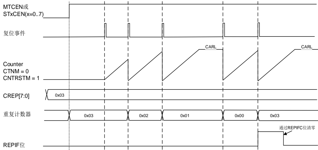
图 25-8. 单脉冲模式下，CNTSTM = 1 时重复计数器的动作
