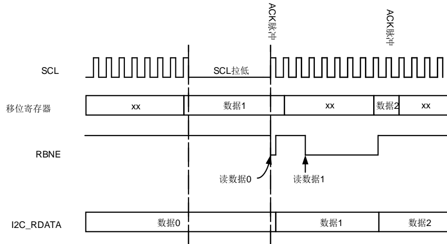
图 28-12. 数据接收
