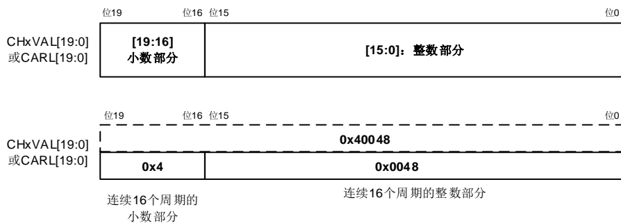
图 23-146. 微调模式：数据格式和寄存器位域
