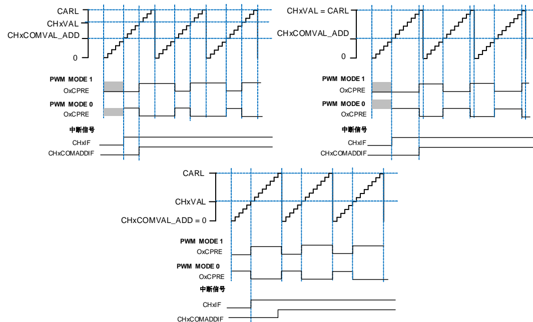
图 23-109. 通道 x 输出 PWM ( CHxVAL > CHxCOMVAL\_ADD )
