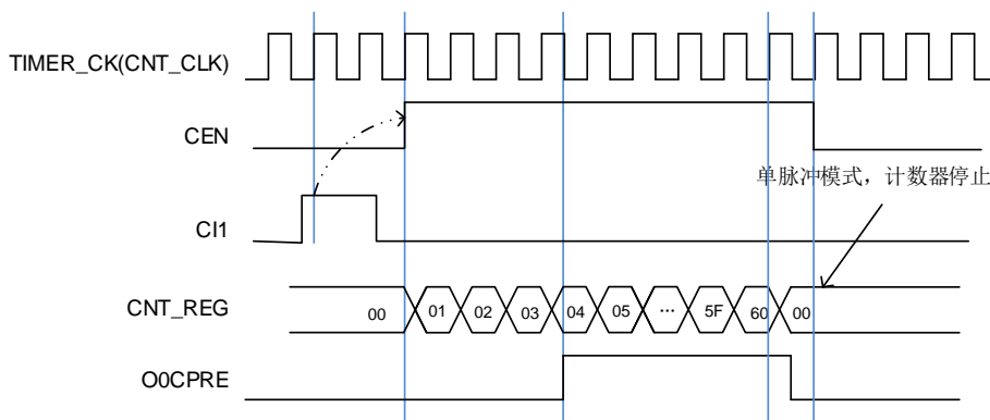
图 23-90. 单脉冲模式， TIMERx_CHxCV = 0x04 ， TIMERx_CAR = 0x60
