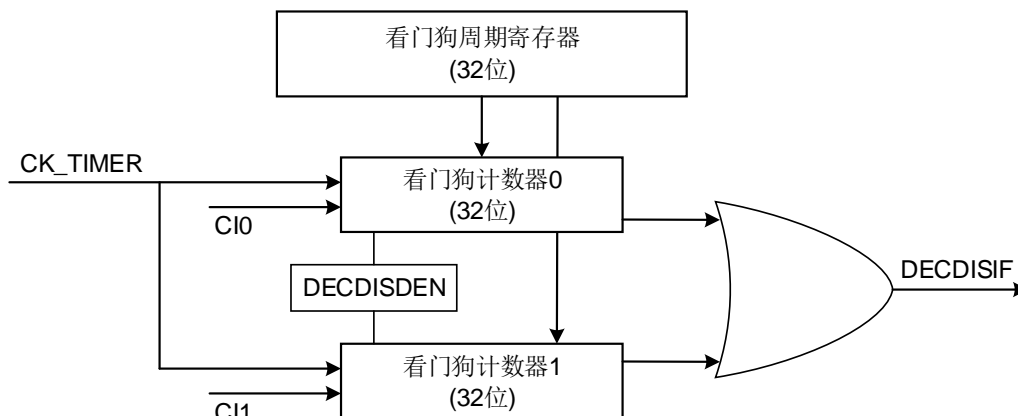
图 23-38. 正交译码器信号断线检测框图
