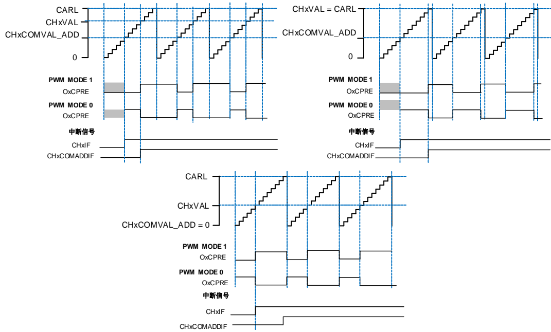
图 23-23. 通道 x 输出 PWM (CHxVAL > CHxCOMVAL_ADD)
