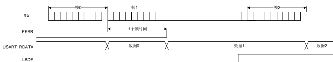
图 27-10. 数据传输过程中检测断开帧
