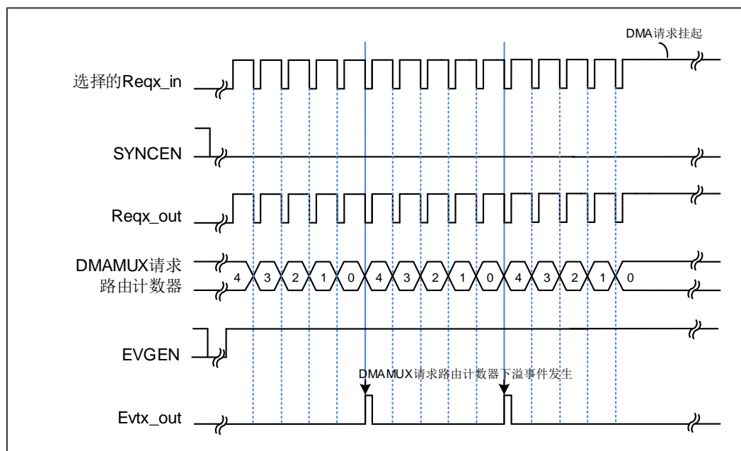
图 9-3. 通道事件输出
