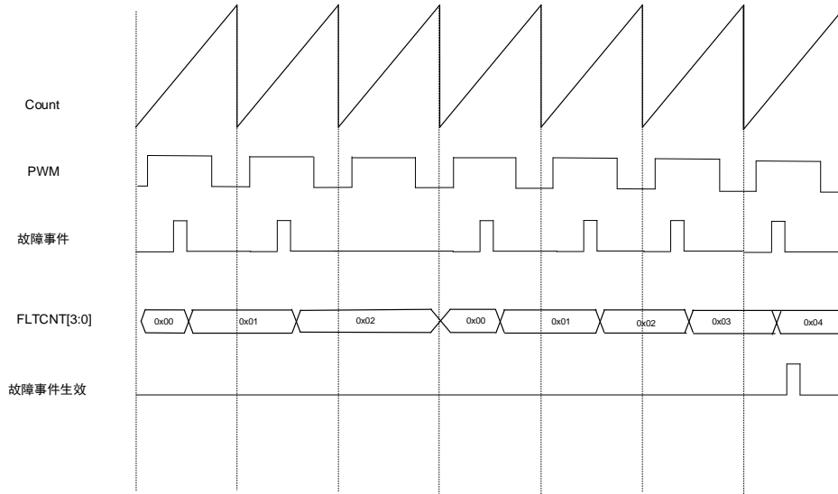
图 25-52. 当 FLT x RST 为 1 和 FLT x CNT[3:0] = 0x03 时故障计数器
