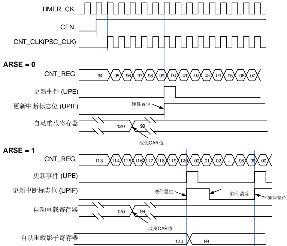
图 23-145. 向上计数时序图，在运行时改变 TIMERx_CAR 寄存器的值
