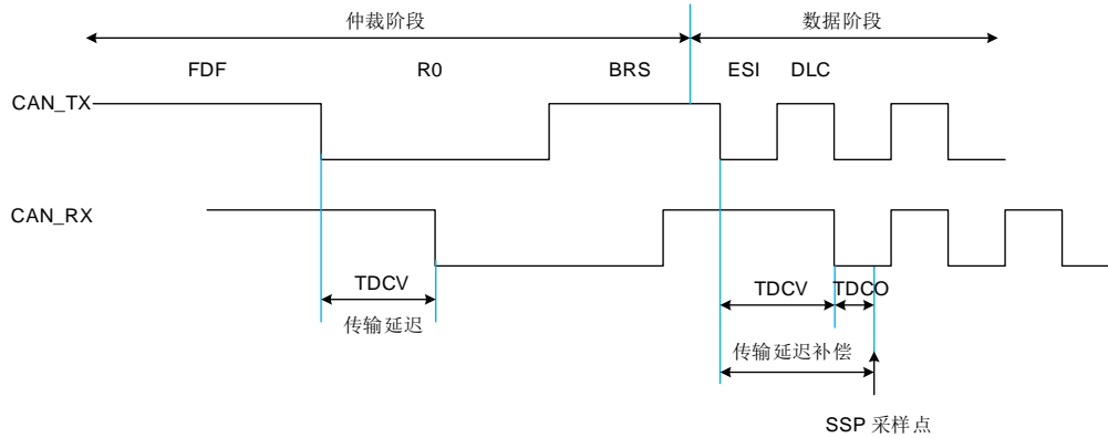
图 29-2. 传输延迟
