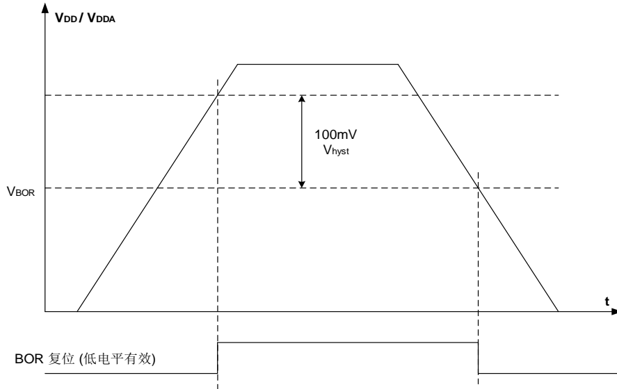
图 3-6. BOR 波形图
