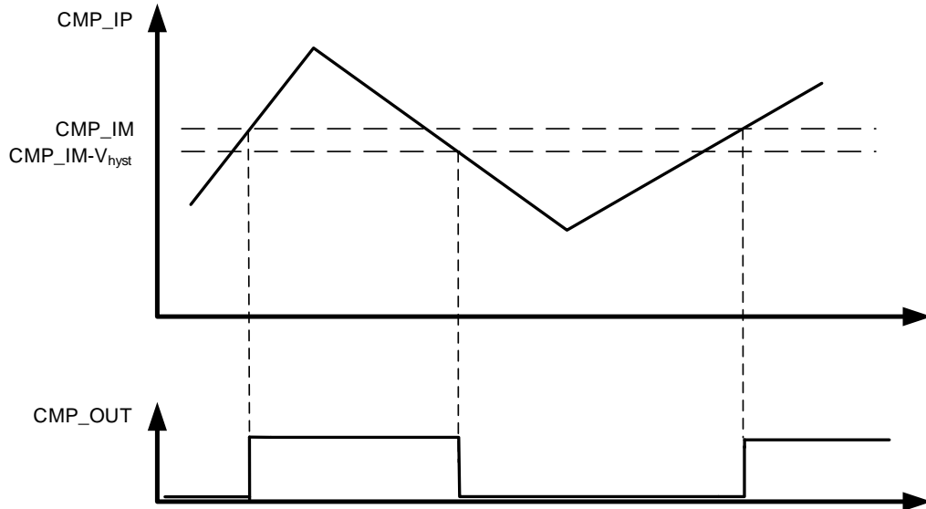
图 19-2. 比较器迟滞
