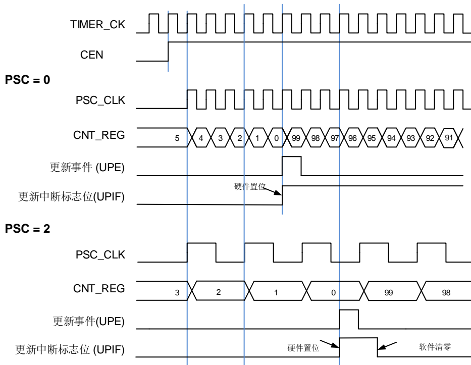
图 23-6. 向下计数时序图, PSC = 0/2
