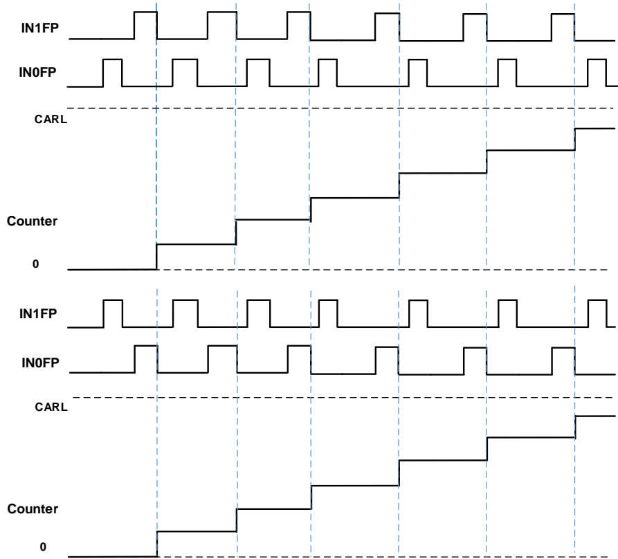
图 24-13. 计数器运行在编码器模式 1（同相）
