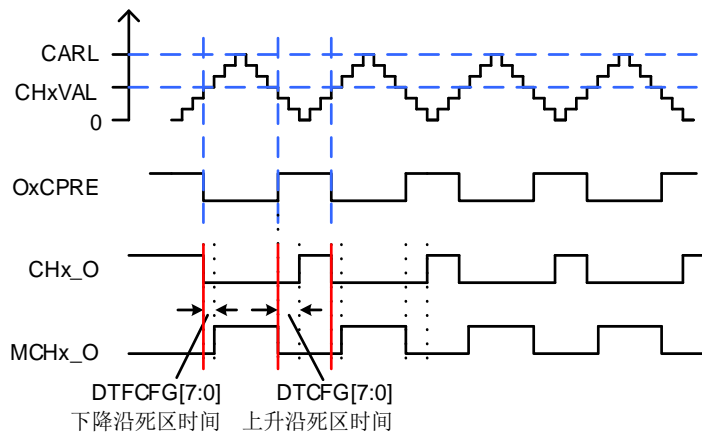
图 23-136.不同死区时间的互补输出（DTDIFEN=1）
