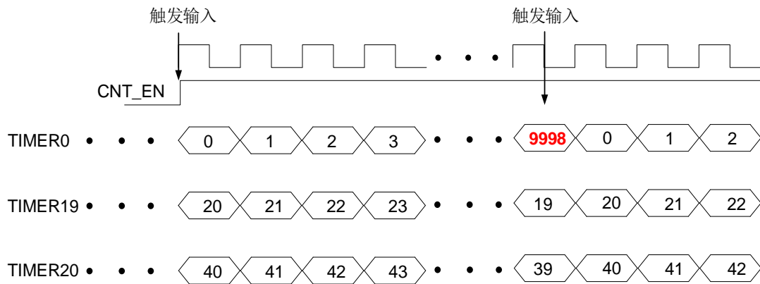
图 23-62. 3 个定时器的相移框图
