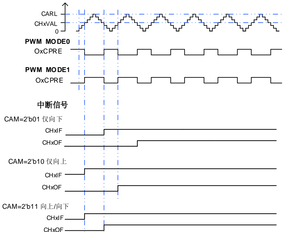
图 23-18. CAPWM 时序图
