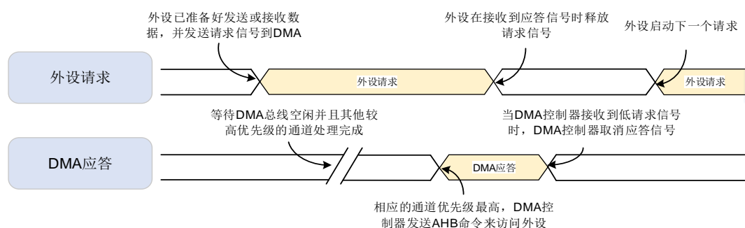
图 8-2. 握手机制
