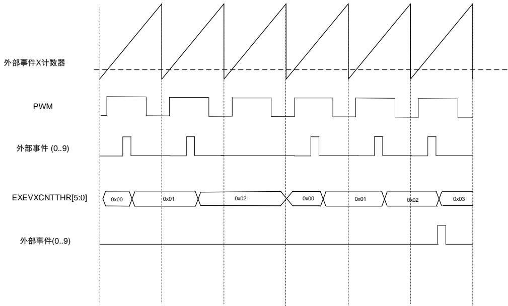
图 25-44. 当 EXEVXCEN 为 1 和 EXEVXCNTTHR[5:0]为 2 时外部事件 X 计数器
