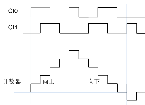
图 23-37. CI0FE0 极性反相的译码器接口模式下的例子
