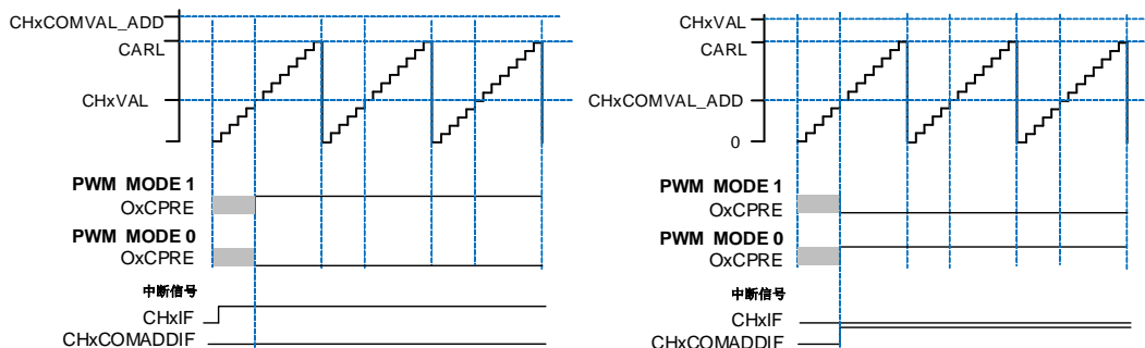
图 23-110. 通道 x 输出 PWM (CHxVAL 或 CHxCOMVAL_ADD > CARL)
