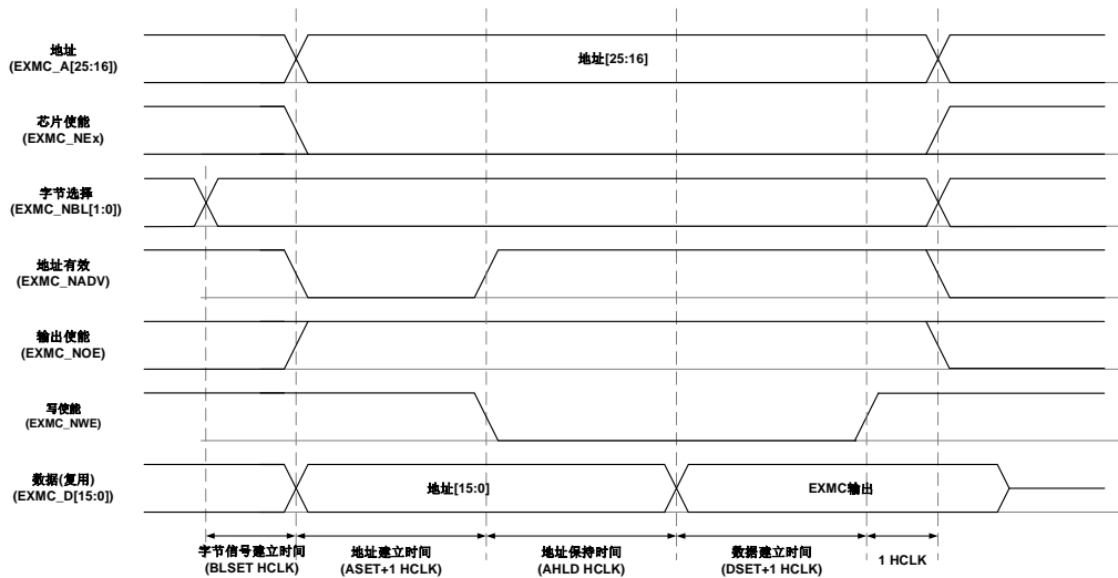
图 33-16. 复用模式写时序
