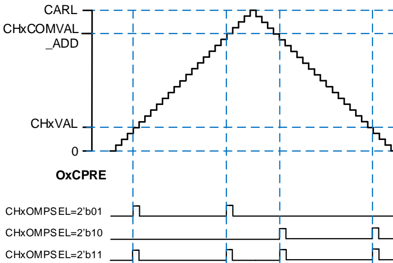
图 23-28. 中央对齐模式下 CHx_O 输出脉冲 (CHxOMPSEL ≠ 2'b00)
