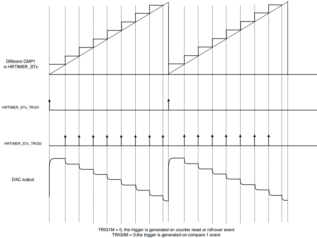
图 25-57. 当 TRIG0M= 0 和 TRIG1M = 0 时 DAC 触发
