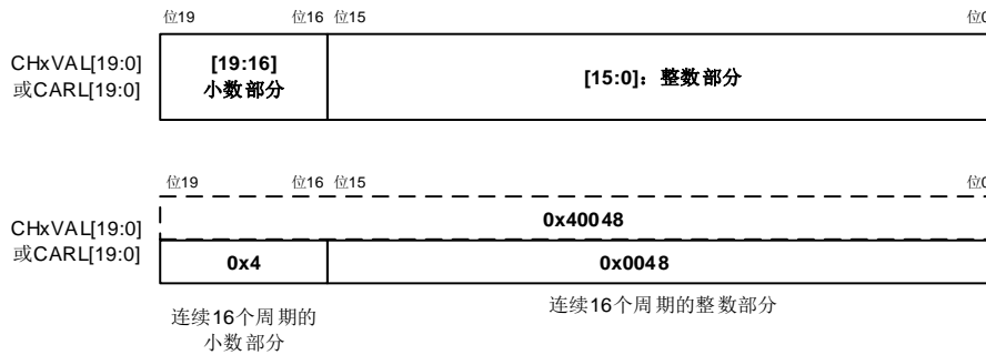
图 23-19. 微调模式: 数据格式和寄存器位域
