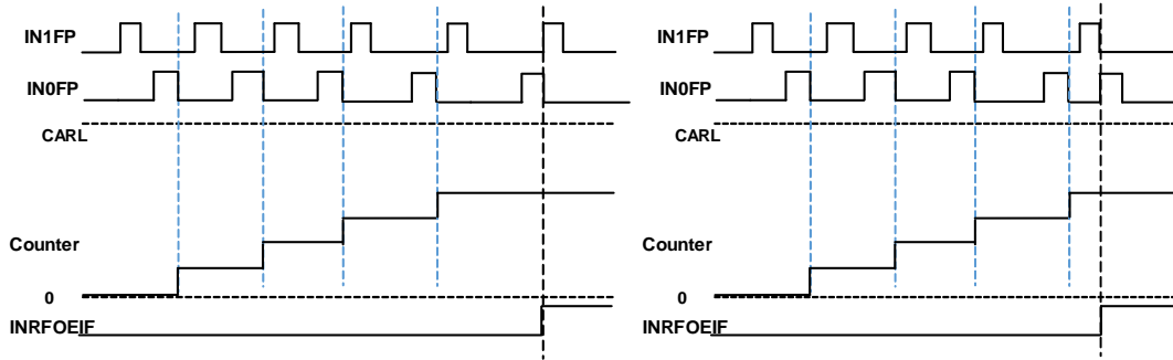
图 24-16. 计数器运行在编码器模式 1 (同相, INRFOEIF)
