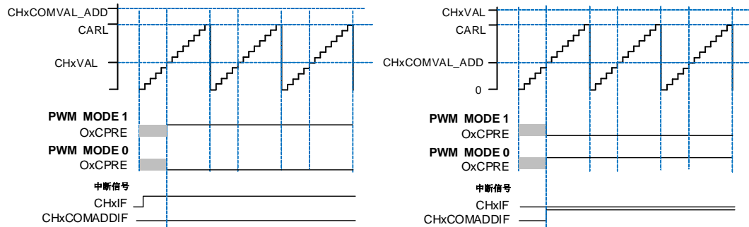
图 23-24. 通道 x 输出 PWM (CHxVAL 或 CHxCOMVAL_ADD > CARL)
