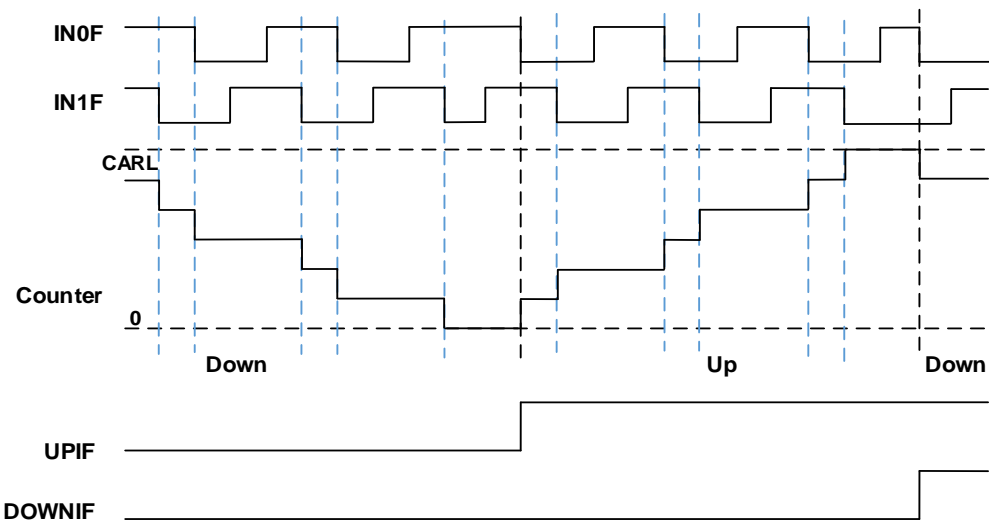
图 24-12. 计数器运行在编码器模式 0（下降沿计数）
