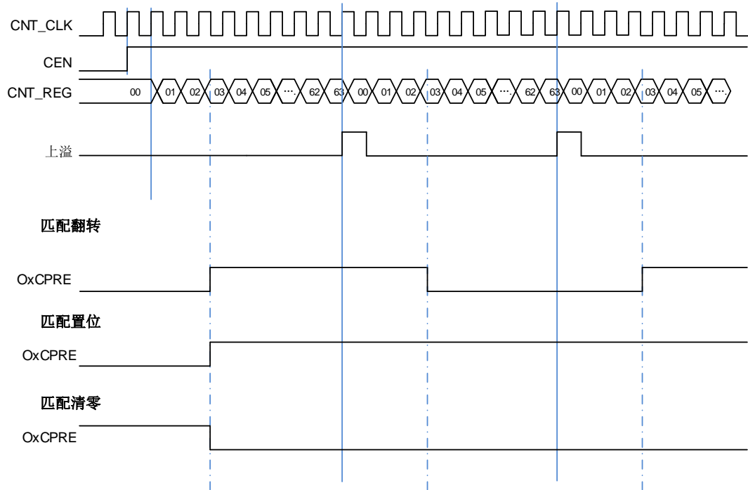
图 23-16. 三种输出比较模式
