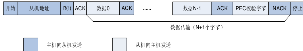
图 28-23. SMBus 主机接收器和从机发送器通信流程
