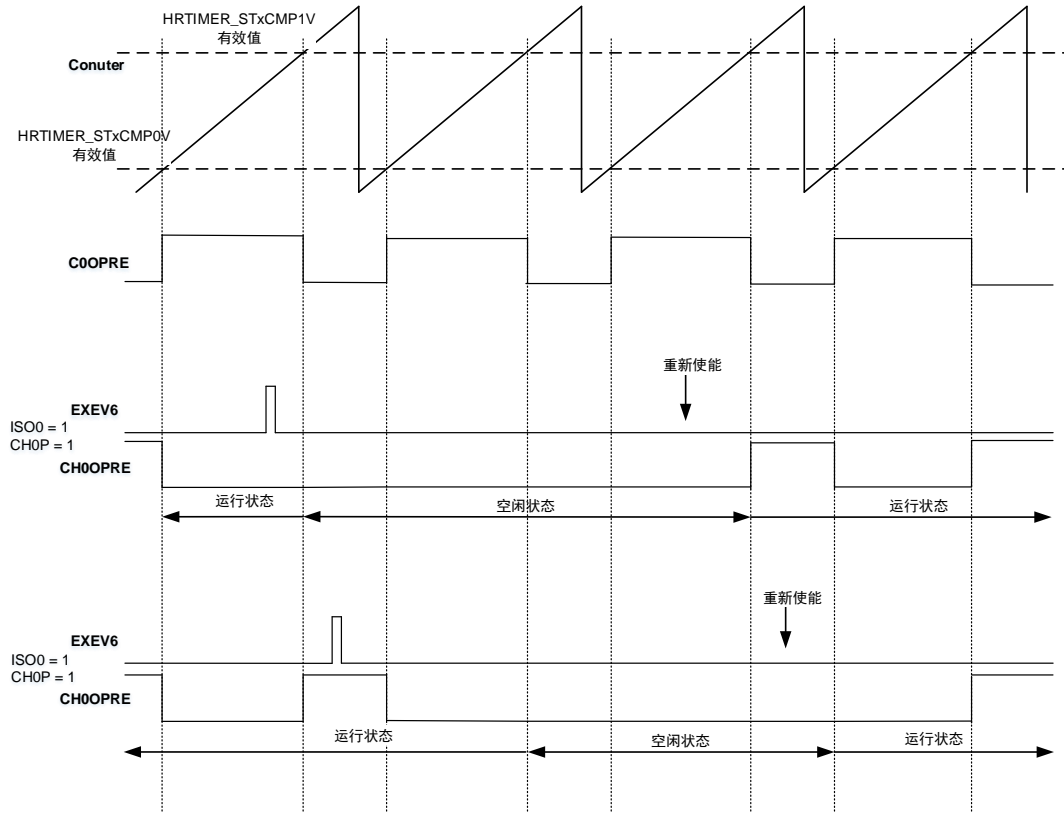
图 25-37. 延迟空闲模式, ISO0 = 1 和 CHOP = 1
