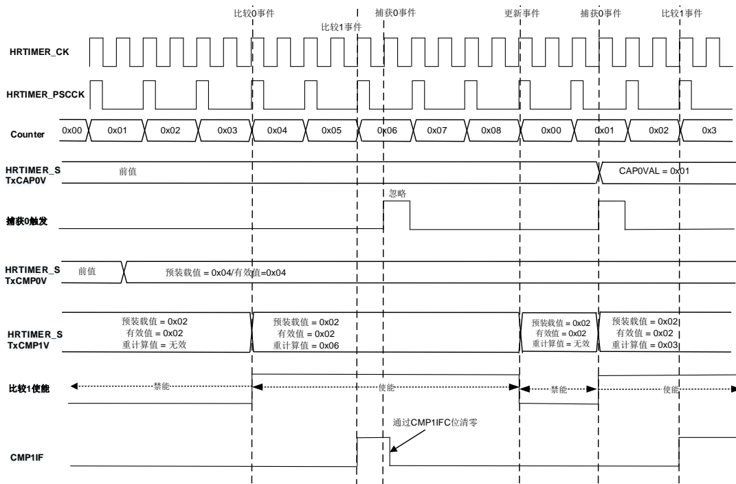
图 25-15. 比较 1 延迟模式 1
