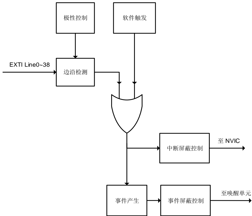
图5-1. EXTI框图
