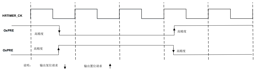
图 25-27. 高分辨率 OXPRE 波形
