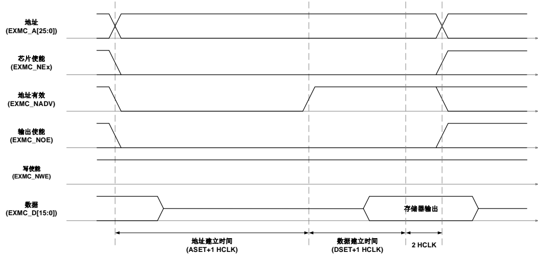
图 33-9. 模式 2 写时序
