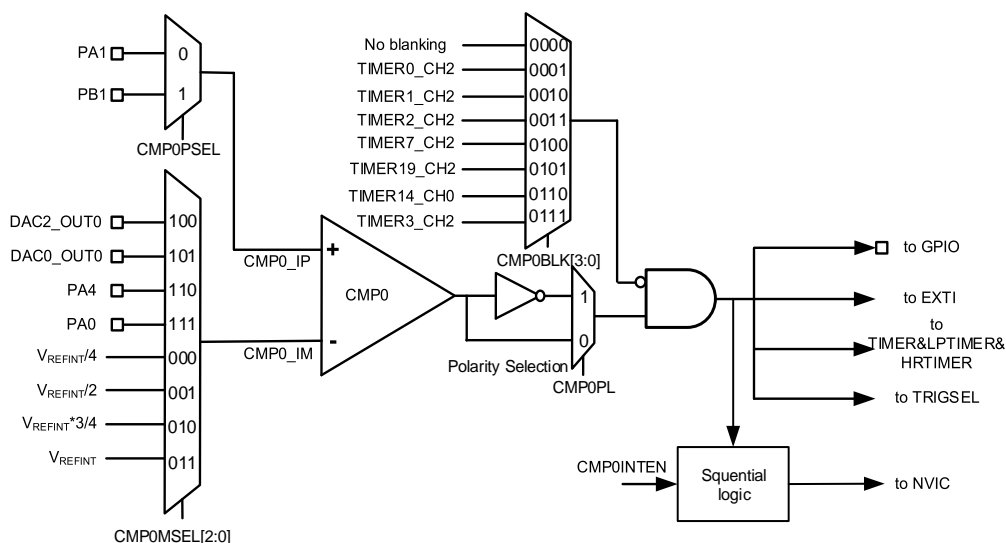
图 19-1.比较器框图
