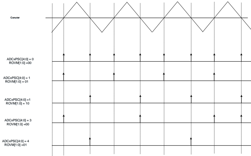
图 25-55. 中央对齐计数模式下 ADC 触发分频
