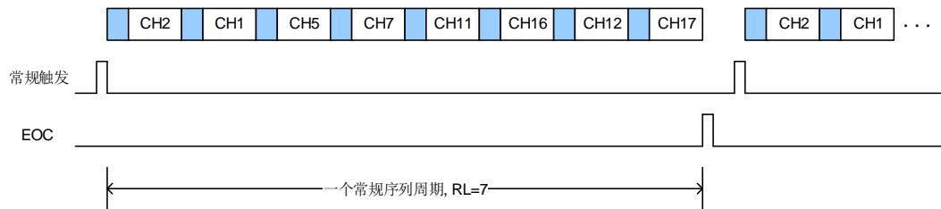
图 17-4. 扫描转换模式，且连续转换模式失能
