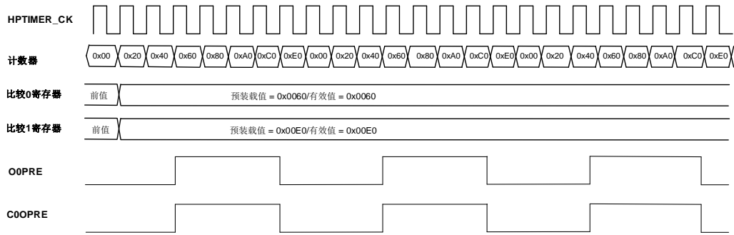
图 25-29. 常规模式下的 C0OPRE 波形
