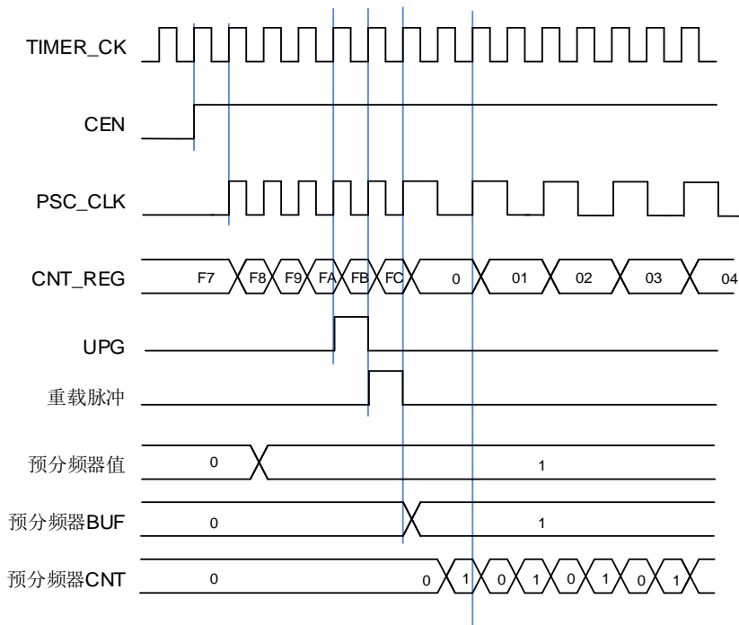
图 23-143. 当预分频器的参数从 1 变到 2 时, 计数器的时序图
