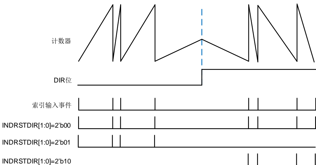
图 23-43. 索引信号和计数器复位事件的关系
