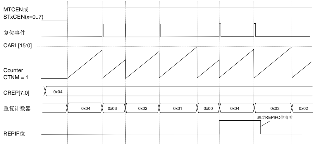
图 25-7. 单脉冲模式下，CNTRSTM = 0 时重复计数器的动作 显示了单脉冲模式下，CNTRSTM = 0 时重复计数器的运行情况。
