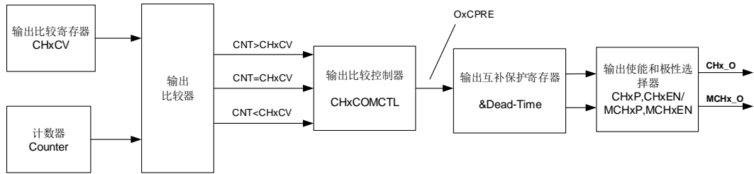
图 23-15. 输出比较逻辑（当 MCHxMSEL = 2'b11 时，x = 0,1,2,3）
