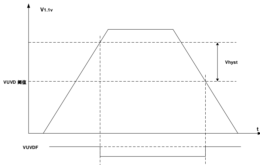
图 3-10. VUVD 波形
