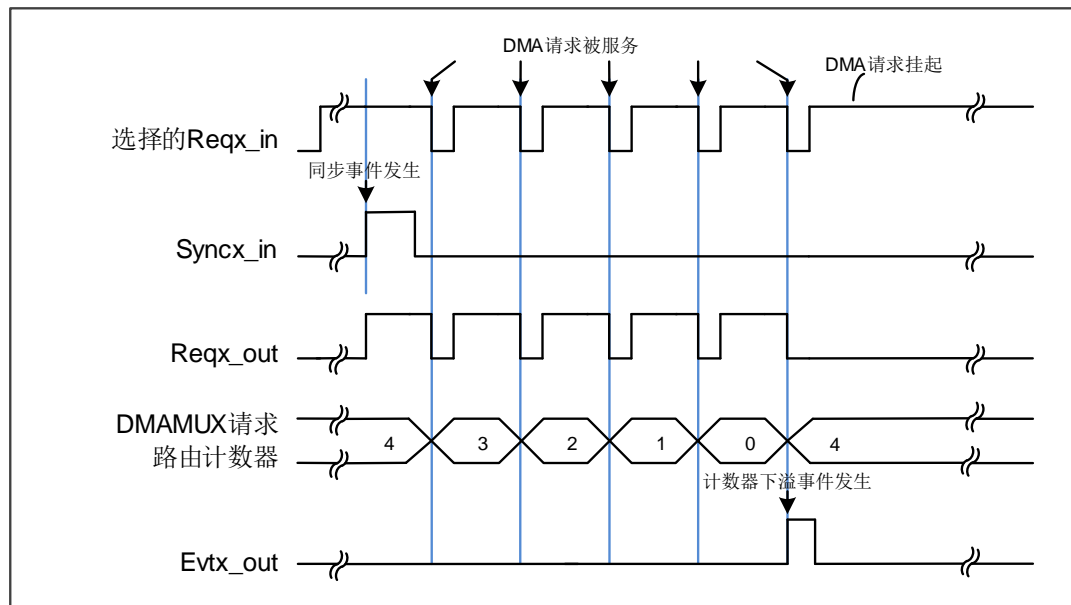
图 9-2. 同步模式
