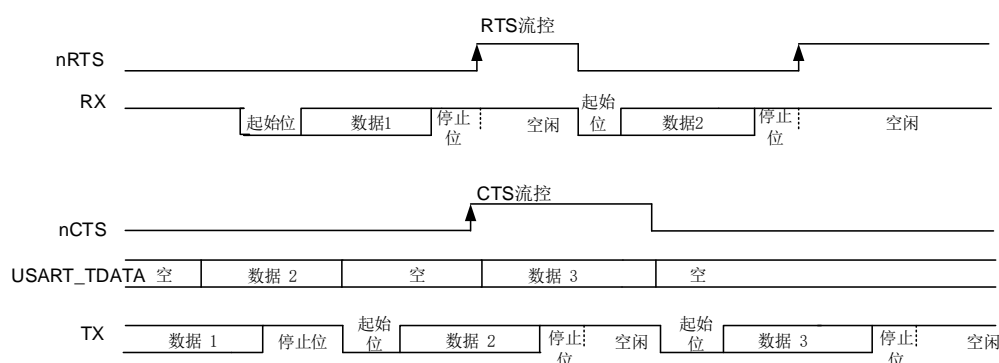
图 27-8. 硬件流控制
