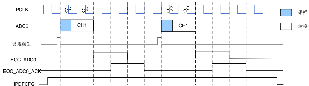
图 17-9. HPDF 与 ADC 模块握手信号示意图
