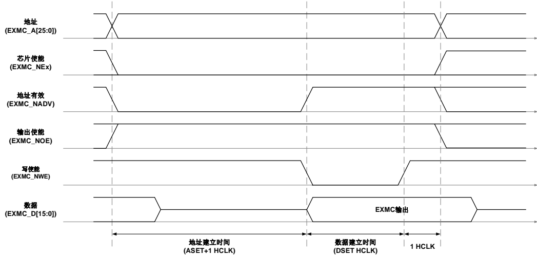
图 33-10. 模式 B 写时序
