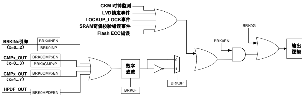
图 23-137. BREAK0 中止功能逻辑图
