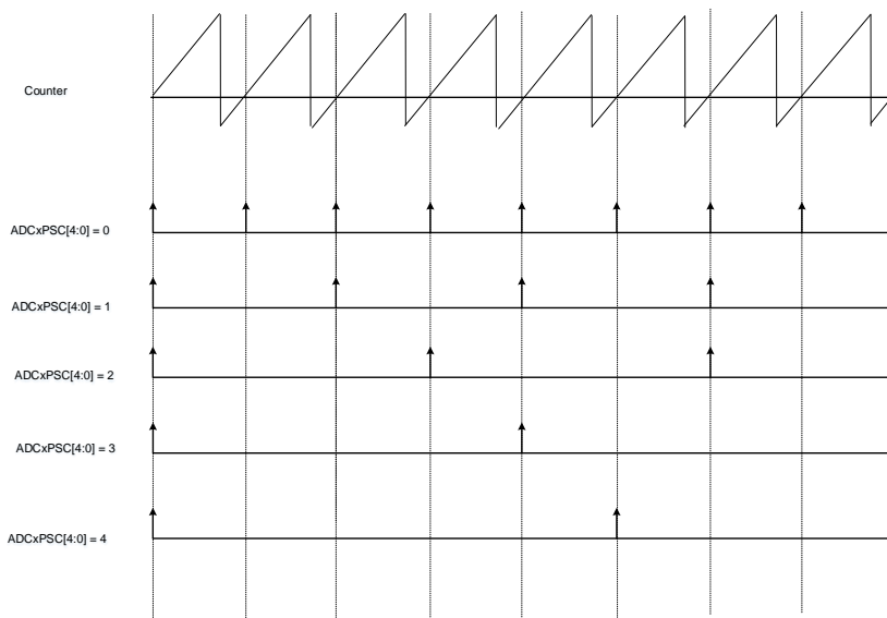
图 25-54. 向上计数模式下 ADC 触发分频
