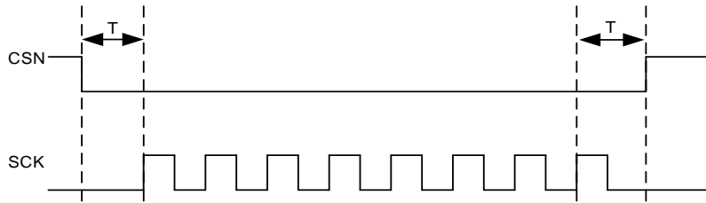
图 31-5. CSN 和 SCK 的行为 (CSNCKM = 0)
