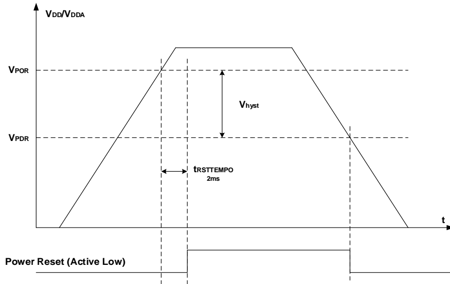
图 3-5. 上电 / 掉电复位波形图
