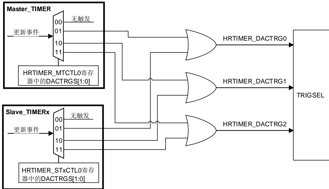
图 25-56. DAC 触发源选择图
