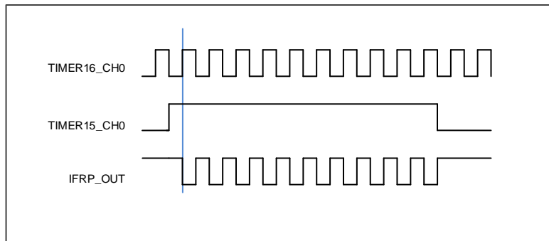
图 26-1. IFRP 输出时序图 1
