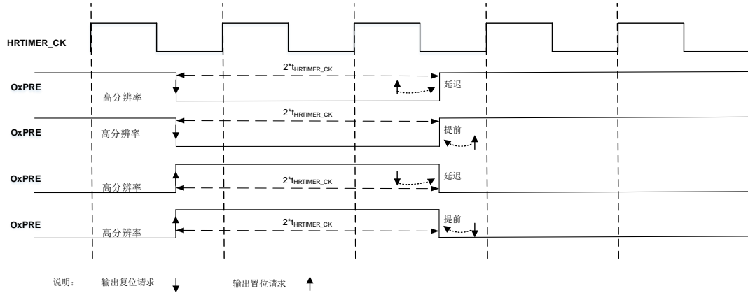
图 25-26. 脉冲宽度为 2 个 t_{HRTIMER\_CK} 周期
