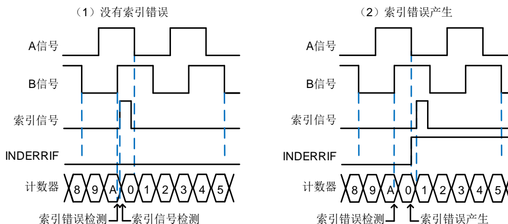
图 23-45. 向上计数模式时的索引错误检测
