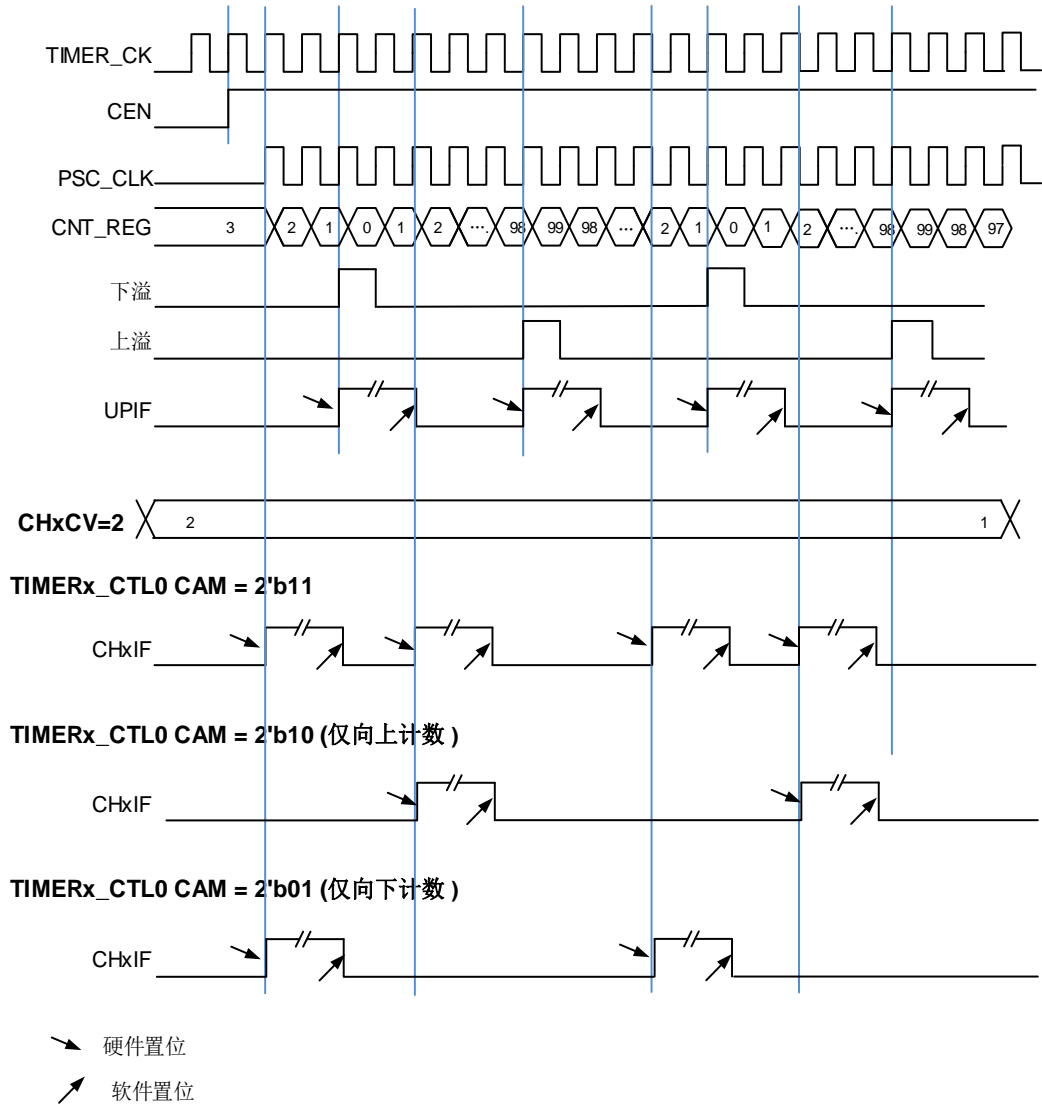
图 23-71. 中央计数模式计数器时序图
