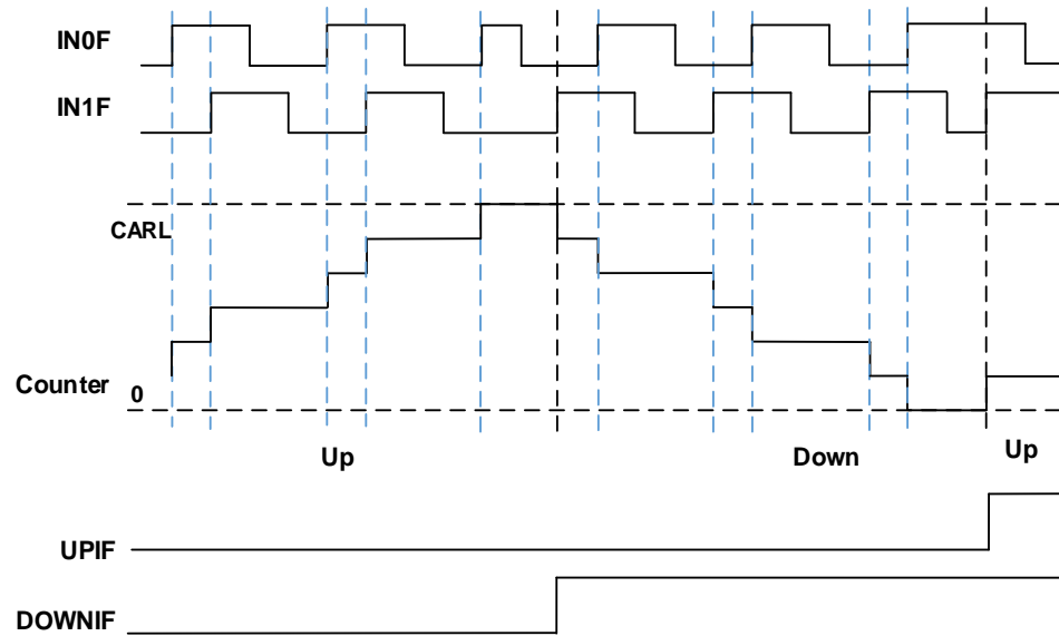
图 24-11. 计数器运行在编码器模式 0（上升沿计数）
