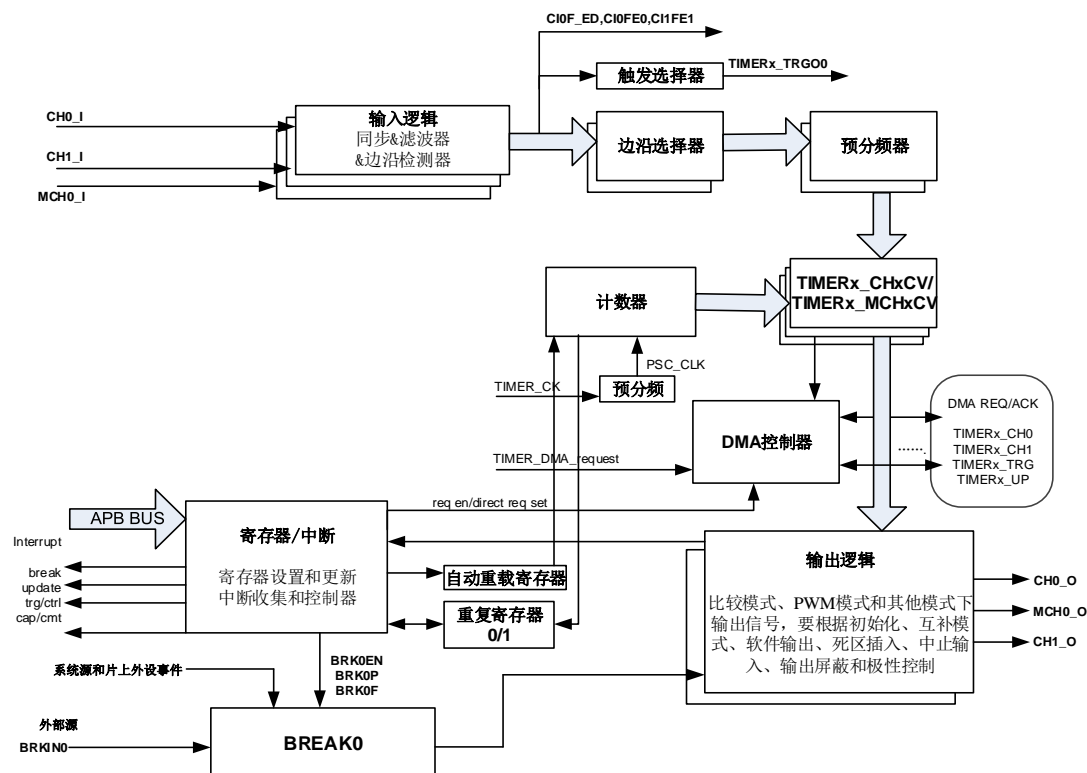
图 23-92. 通用定时器 L3 结构框图
