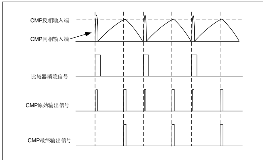
图 19-3. 比较器的输出消隐
