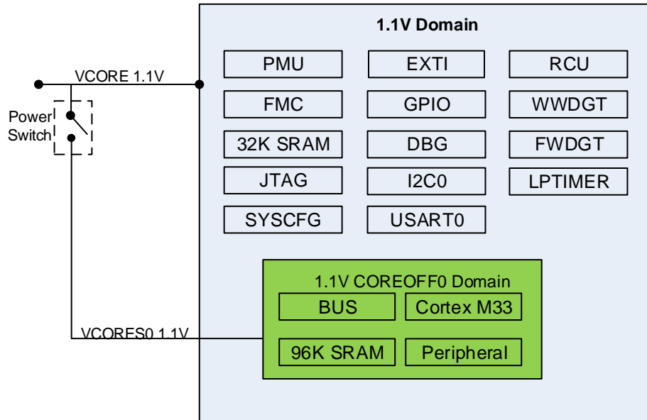
图 3-2. 1.1V 电源域概览
